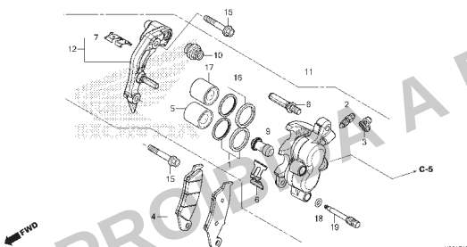
C-12 Cáliper do Freio Dianteiro
