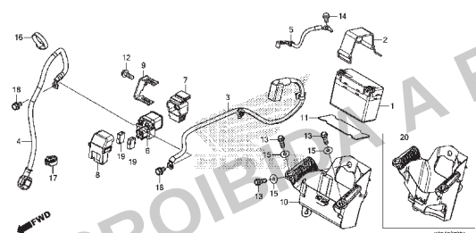
C-37 Bateria
