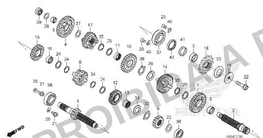
M-17 Transmissão
