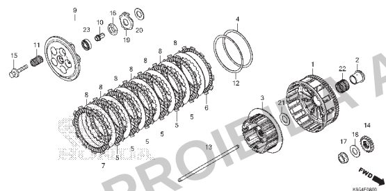
M-8 Embreagem
